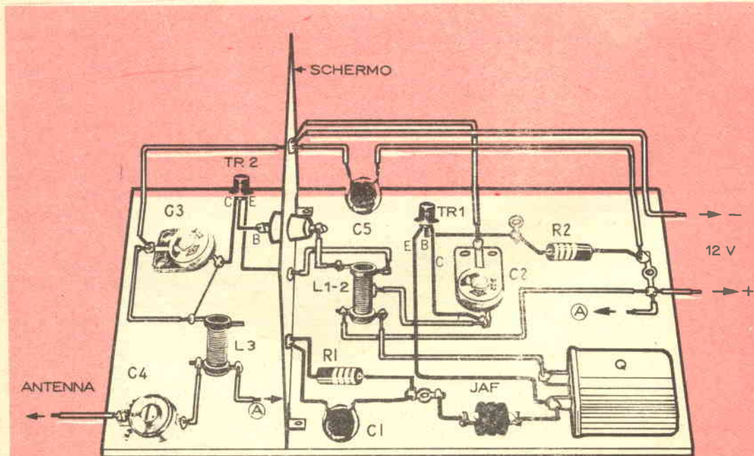
SCHEMA PRATICO
