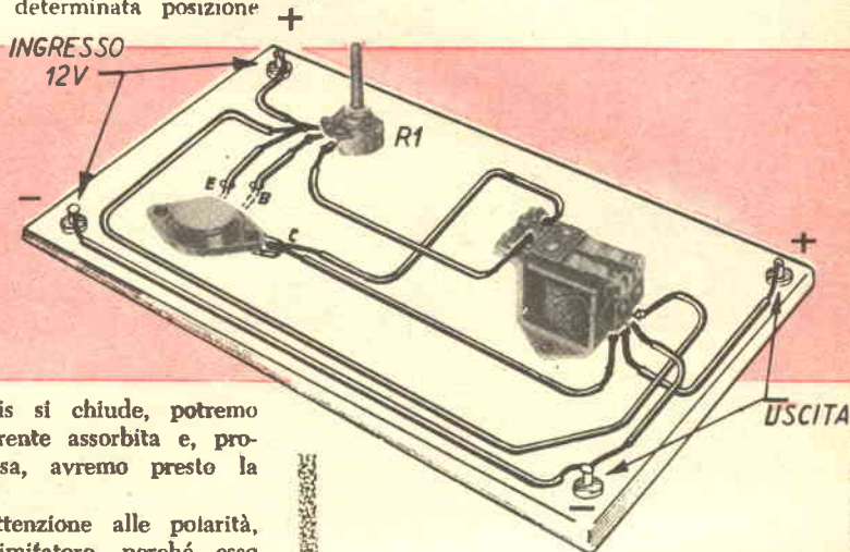
SCHEMA PRATICO
